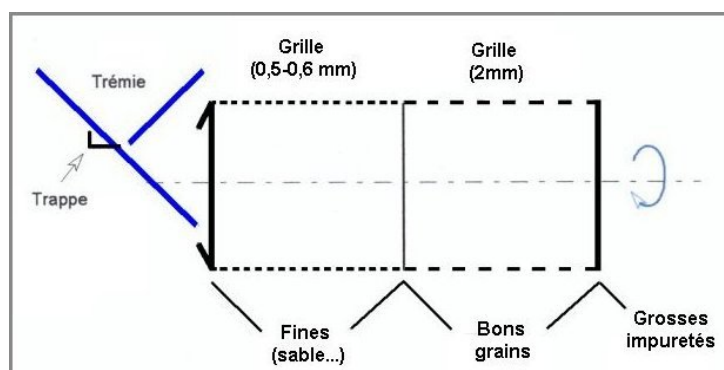
Schéma du crible rotatif (© Cruz et al. , 2011)
